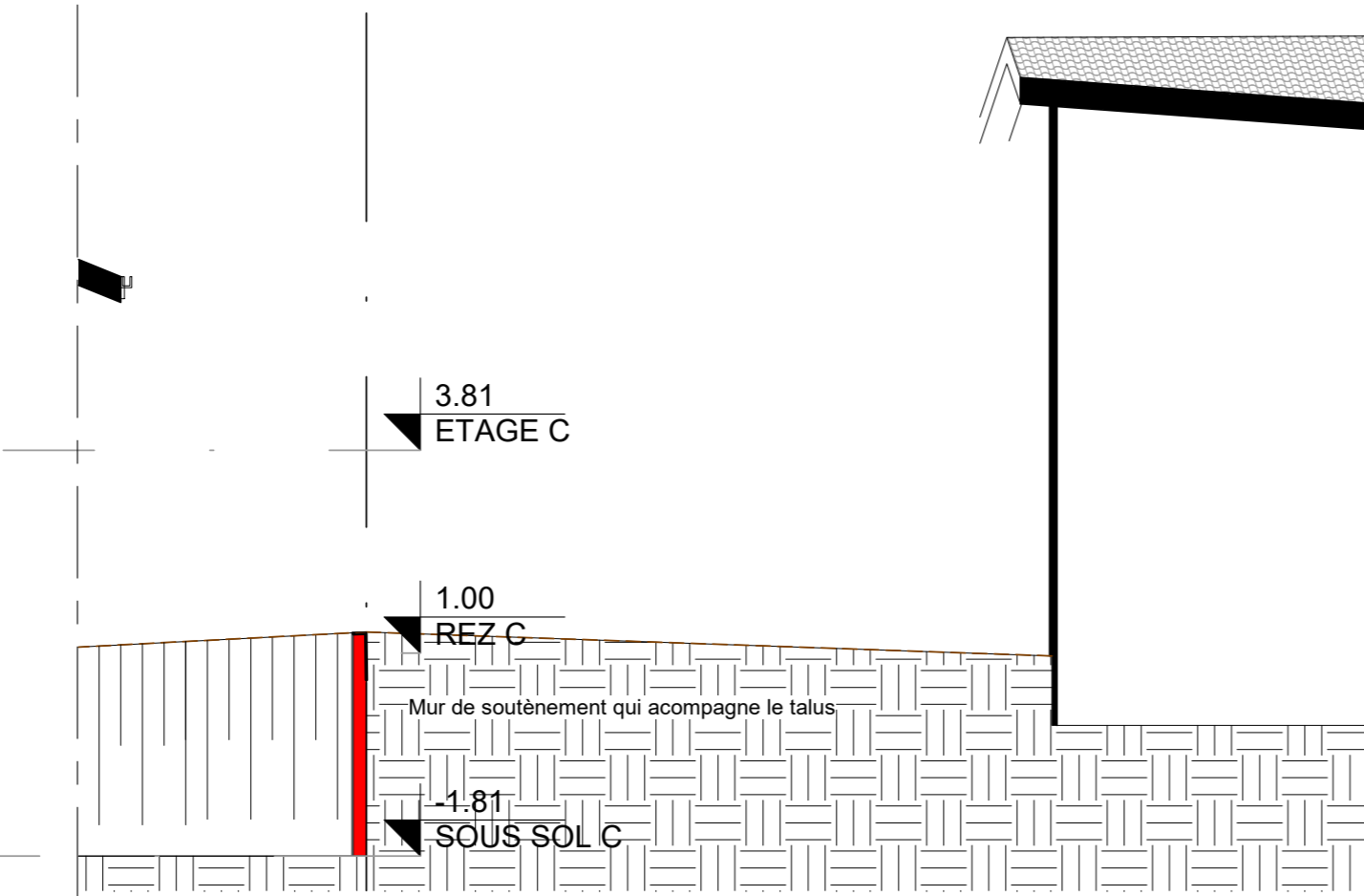
3 Coupe 2 1 : 100
